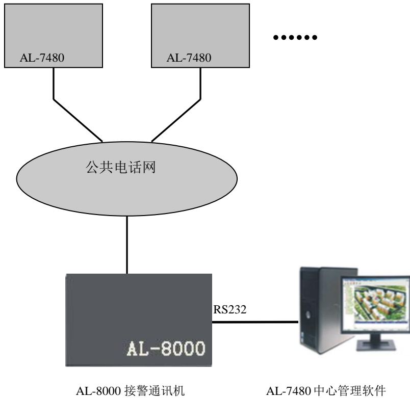
AL-7480 通过电话网络与中心连接示意图
