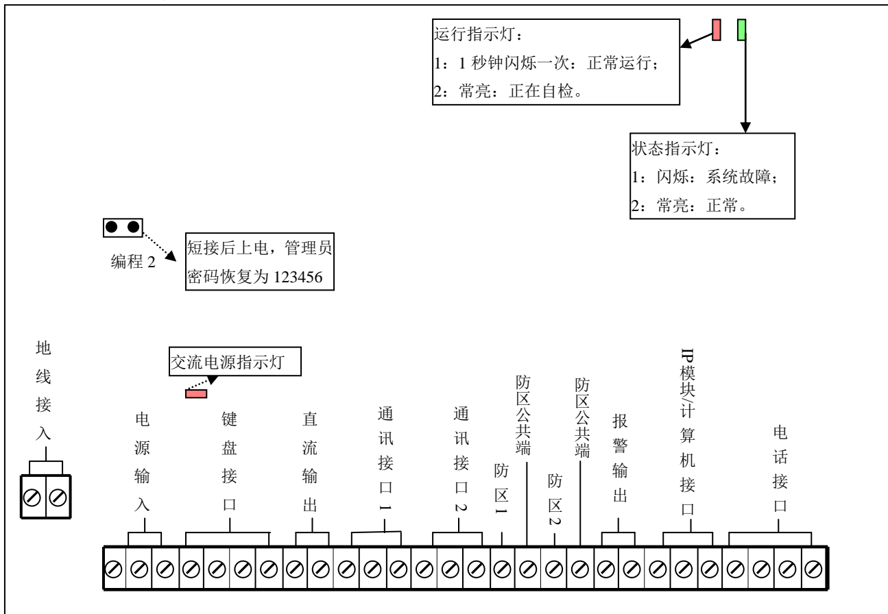
AL-7480 报警主机端口示意图
