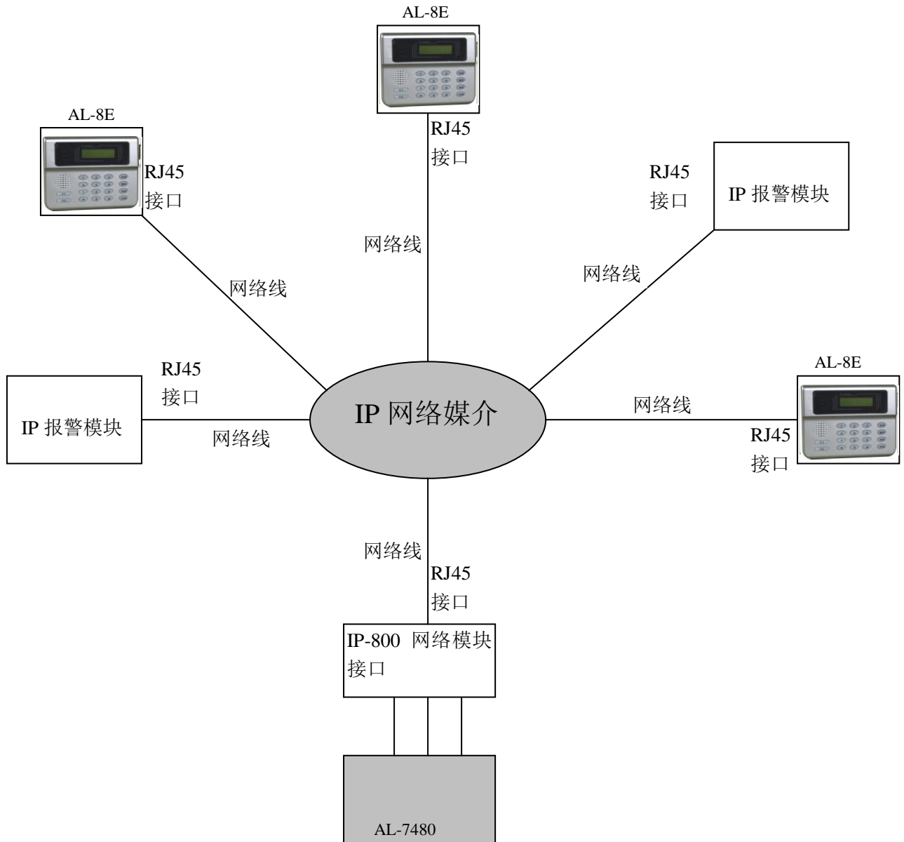
AL7480 与网络接警设备连接示意图
