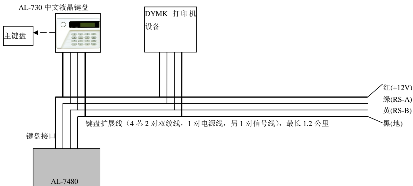
AL-7480 与主键盘、打印设备连接示意图
