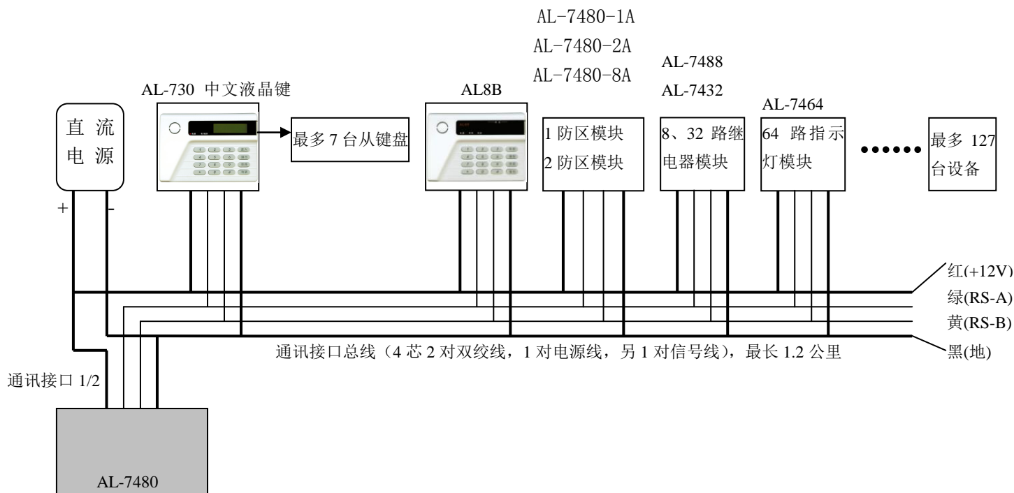
AL-7480 与总线设备连接示意图
